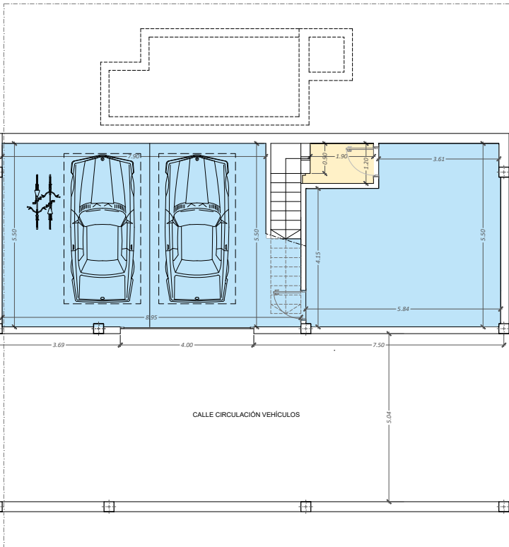
PLANTA SOTANO
