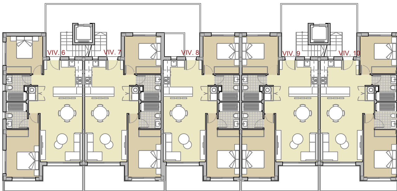
PLANTA PISO
