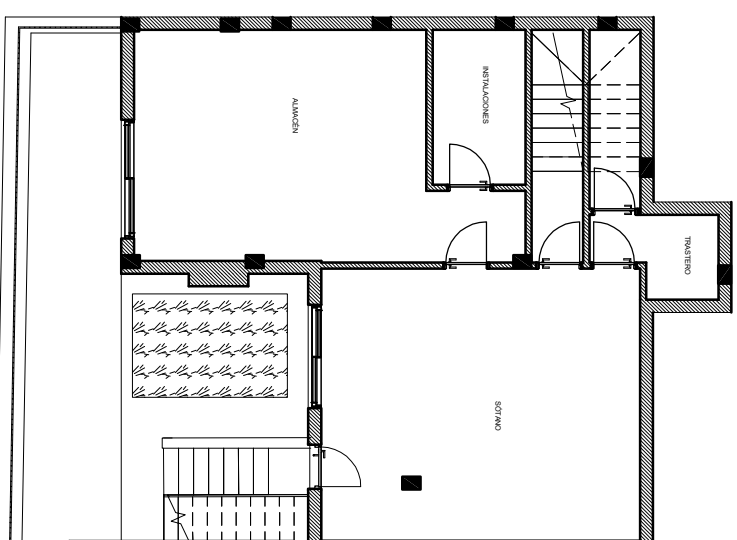
PLANTA SEMISÓTANO
